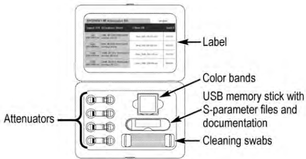
检定为 DPO7RFK1-1.85 mm 的衰减器套件
