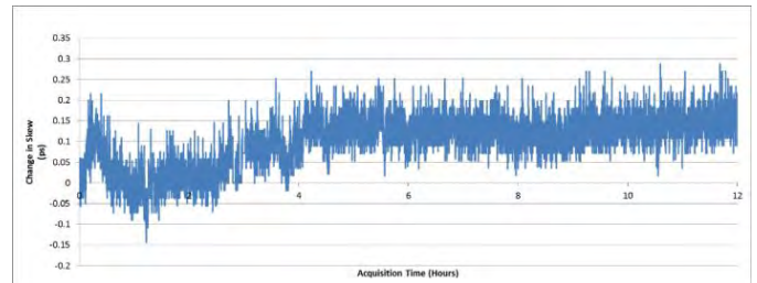
DPO77002SX 系统通道间时延随时间变化。
